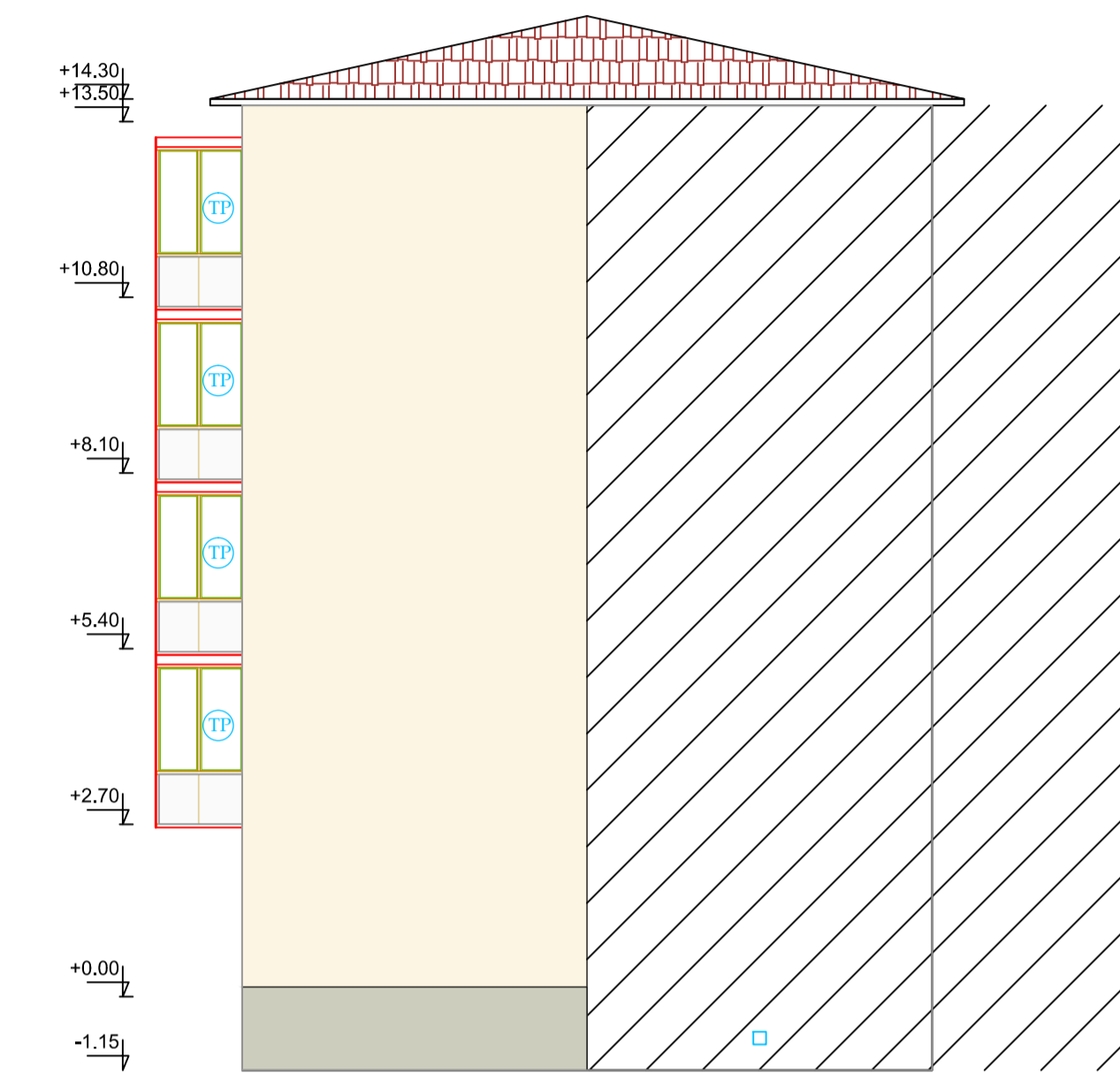
FATADA LATERALA DREAPTA PROPUSA
